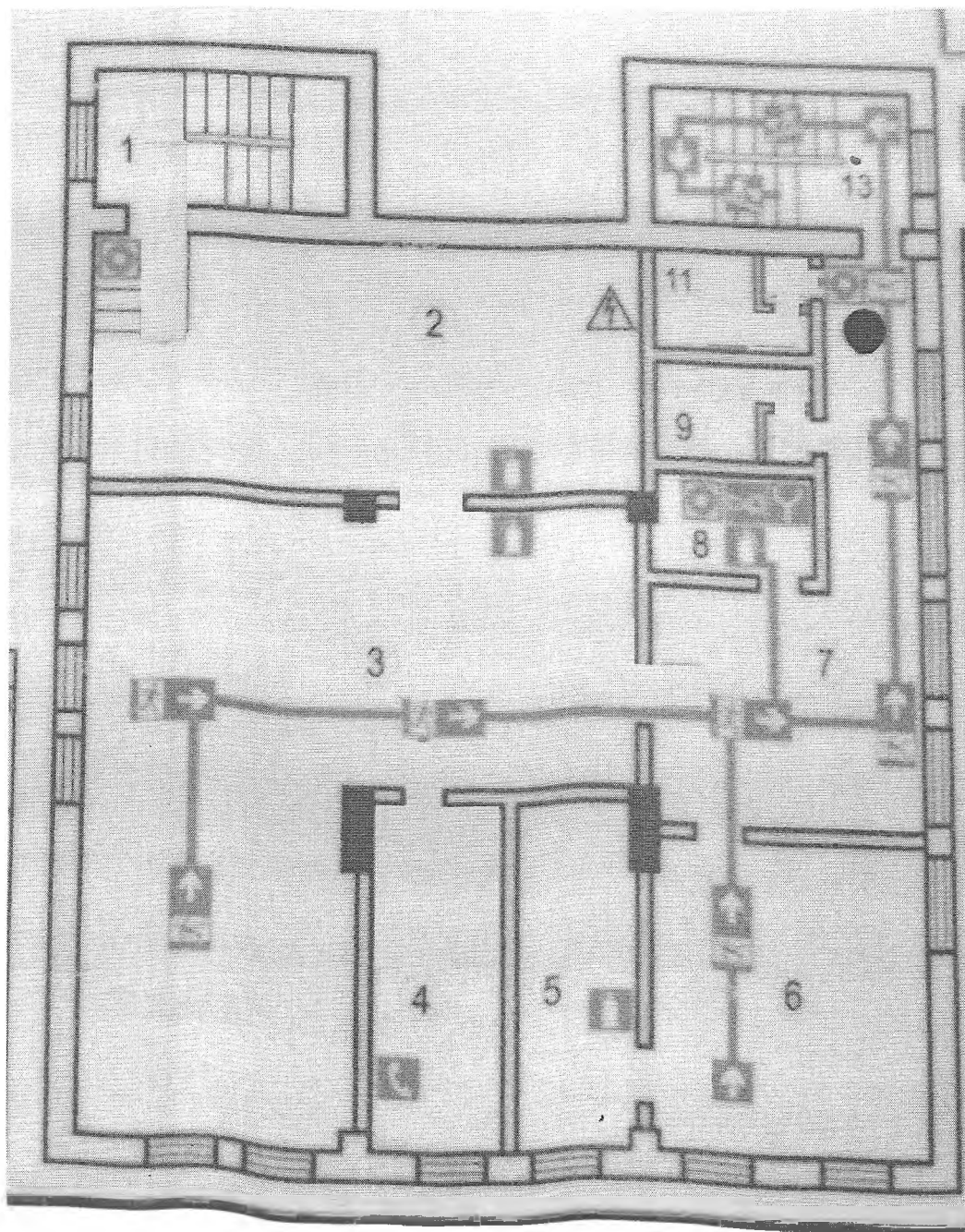
Маршрут (схема) движения инвалидов и других МГН на объекте
